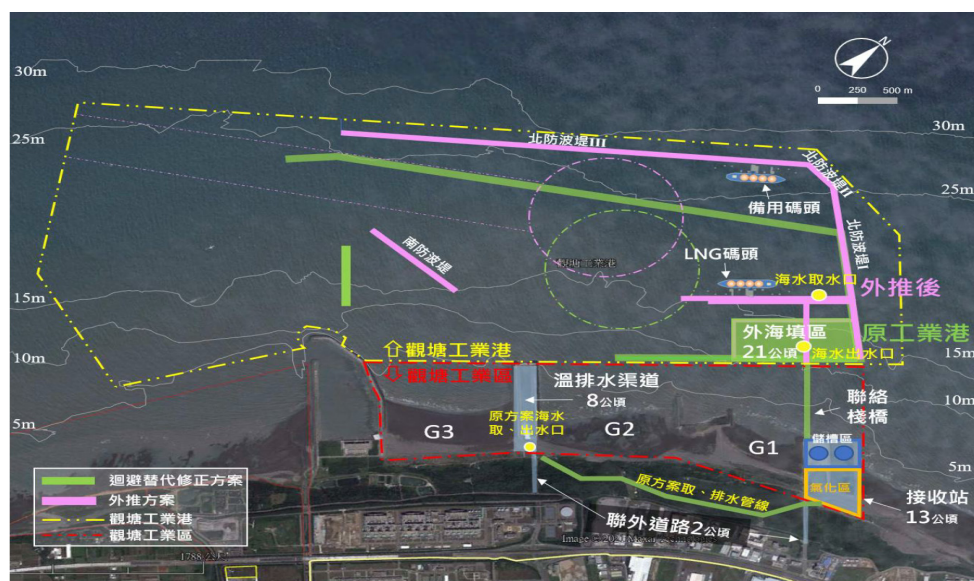
外推方案示意圖
